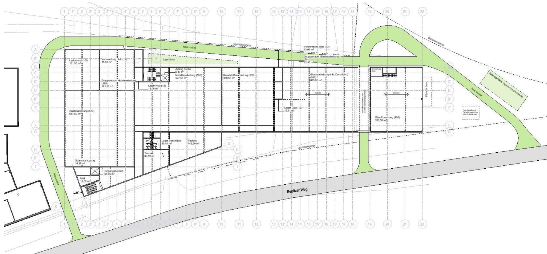
Errichtung neue Umfahrt für Anlieferung und Feuerwehr und Außenlagerflächen
